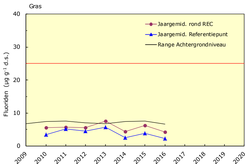
Figuur 10 Trendmatig verloop van het gemiddelde fluoridengehalte in gras ( \mu\text{g g}^{-1} \text{ d.s.} ) in de directe omgeving van de REC en het referentiepunt, buiten de directe invloedssfeer van de installatie. De rode lijn geeft de adviesnorm van 25 \mu\text{g g}^{-1} \text{ d.s.} weer als maximaal toelaatbaar fluoridengehalte in veevoer voor jongvee (VROM, 2001). De zwarte lijnen geven de bandbreedte voor het achtergrondniveau weer (zie Bijlage 1). NB. In 2010 was de REC nog niet operationeel.
