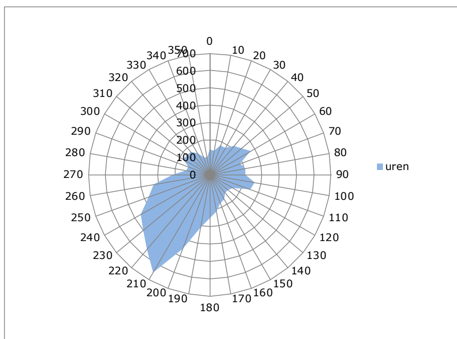
Figuur 3-1 Windroos op basis van metingen van het KNMI weerstation vliegveld Eelde 2016.
