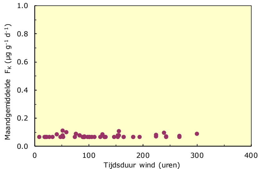
Figuur 7 Fluoridengehalte in kalkpapieren ( F_k ; \mu\text{g g}^{-1} \text{d}^{-1} ) in relatie tot het aantal uren wind per expositieperiode van 28 dagen vanuit de richting van de REC naar de meetpunten rond de installatie.
