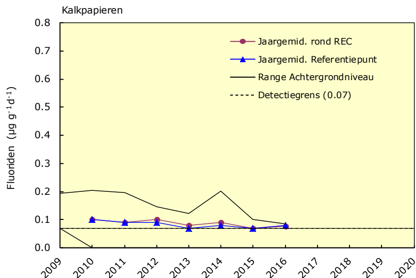
Figuur 8 Trendmatig verloop van het gemiddelde fluoridengehalte in kalkpapieren ( \mu\text{g g}^{-1} \text{d}^{-1} ) in de directe omgeving van de REC en het referentiepunt buiten de directe invloedssfeer van de installatie. De zwarte lijnen geven de bandbreedte van het achtergrondniveau weer (zie Bijlage 1). NB. In 2010 was de REC nog niet operationeel.
